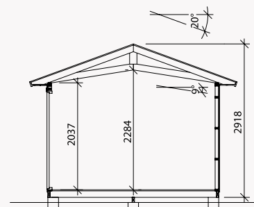
Snitt
