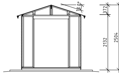
Snitt
