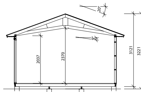
Snitt
